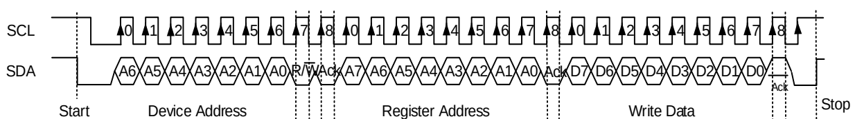
I 2 C Write Byte Cycle
